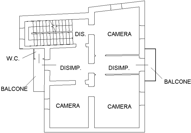
PIANO PRIMO H= 3.75 mt
